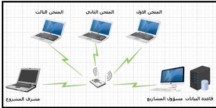
الشكل (3) يوضح التصميم الهيكلي للنظام
