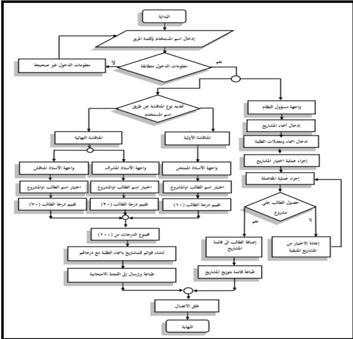
الشكل (4) يوضح المخطط العام للنظام System Flowchart
