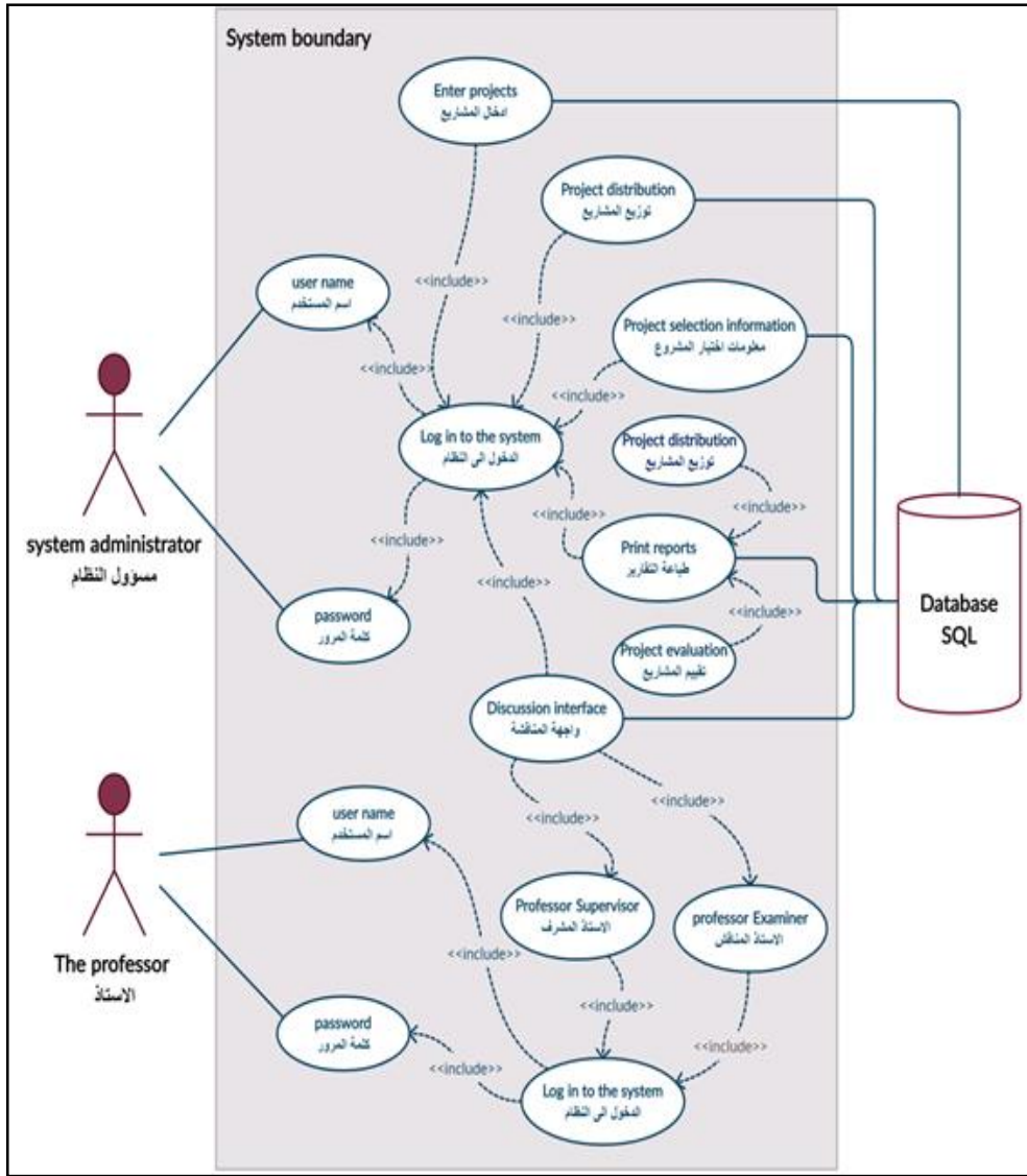
الشكل (2) يوضح مخطط حالة الاستخدام (Use Case Diagram)
