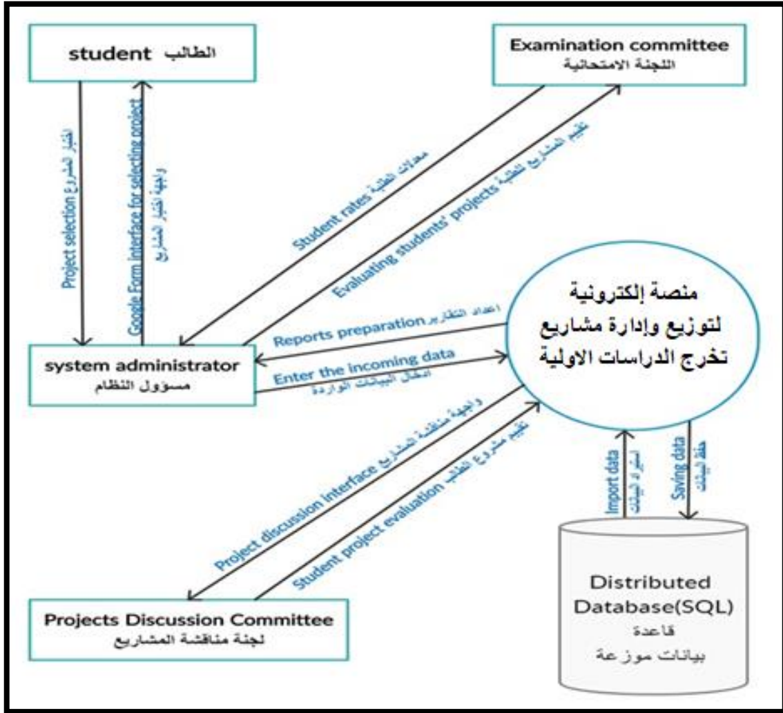
الشكل (1) يوضح مخطط سياق النظام ( System Context Diagram )
